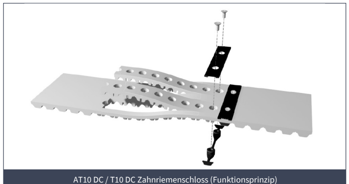
AT10 DC / T10 DC Zahnriemenschloss (Funktionsprinzip)
