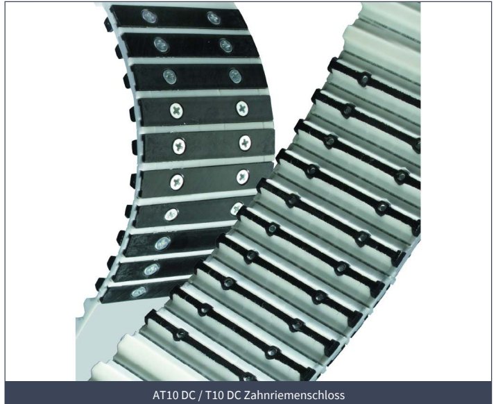
AT10 DC / T10 DC Zahnriemenschloss
