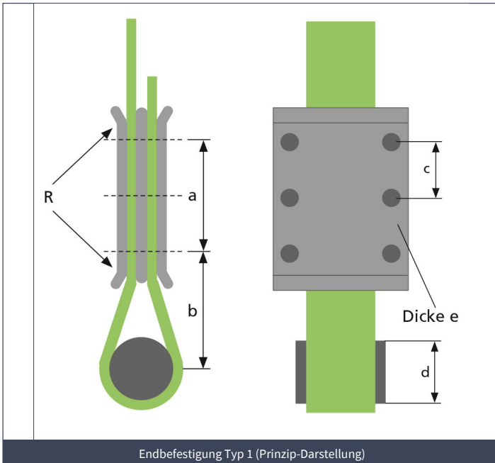
Endbefestigung Typ 1 (Prinzip-Darstellung)
