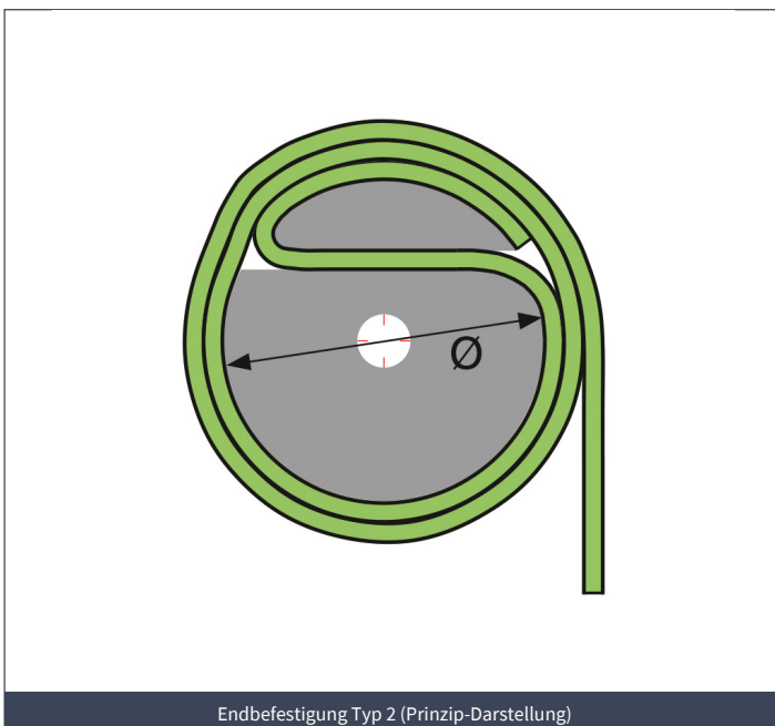
Endbefestigung Typ 2 (Prinzip-Darstellung)
